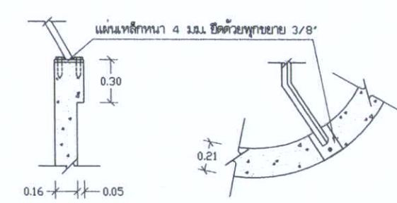
แบบขยายการติดตั้งแอร์เรเตอร์ 1:25
