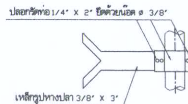
ขยายหลักหางปลา 1:10
