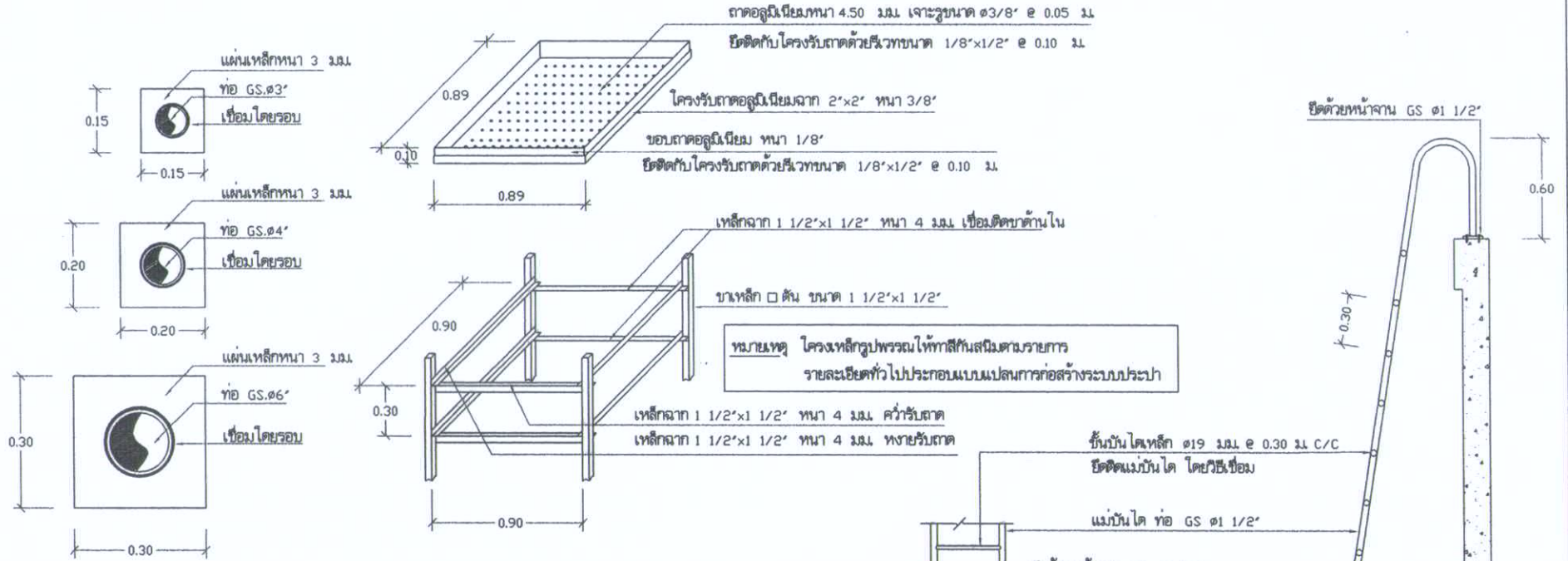
แบบขยายแอร์เรเตอร์ 1:25
