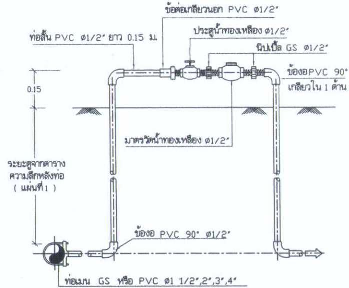
13. การติดตั้งมาตรวัดน้ำ ๑ ๓', ๒' 1:10
